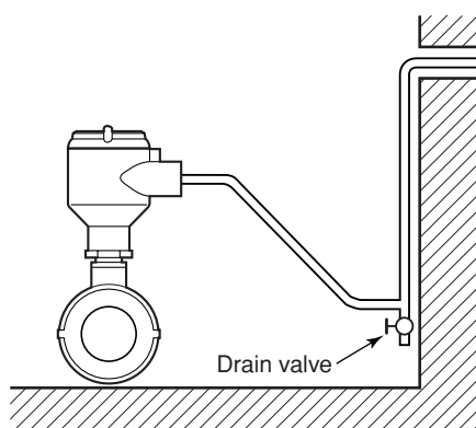
Figure 4.2.7 Conduit Wiring
