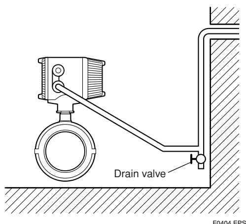
Figure 4.1.4 Conduit Wiring
